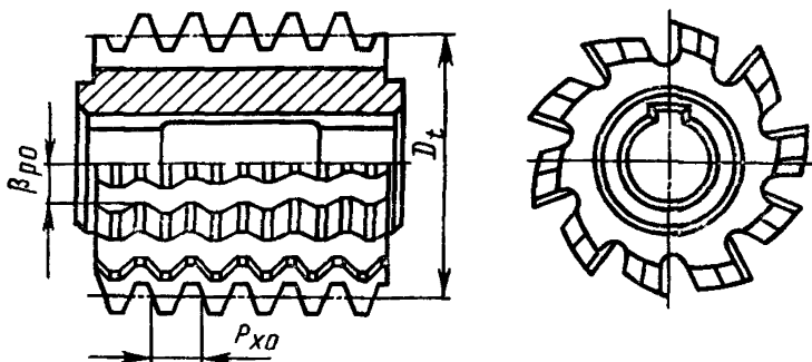
Размеры, мм
